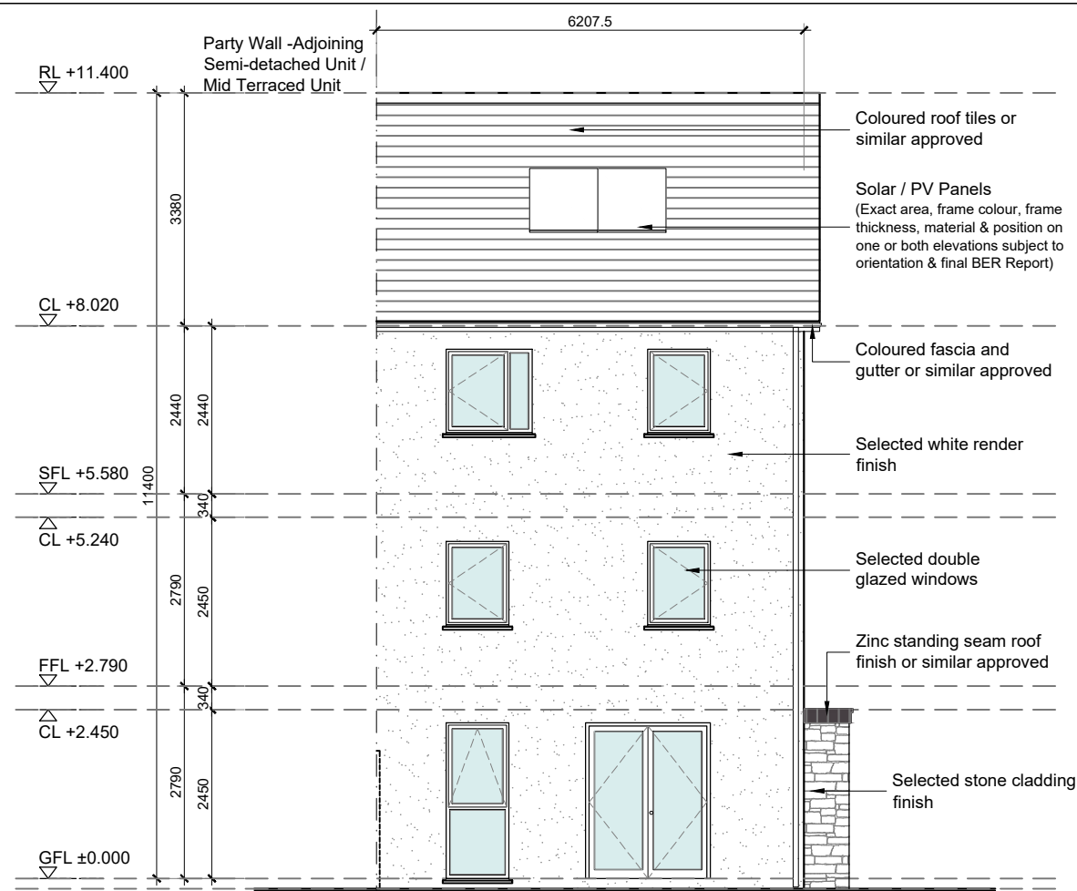
02 Rear Elevation 1:100 @ A3
