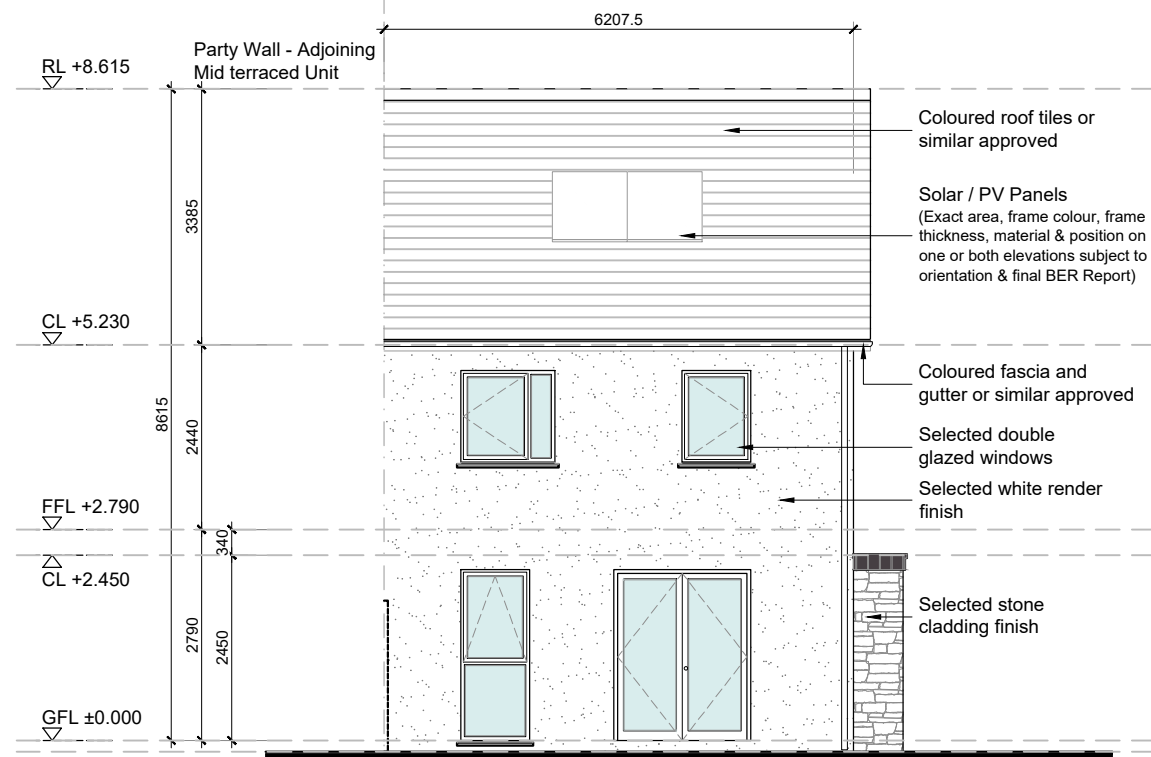
02 Rear Elevation 1:100 @ A3
