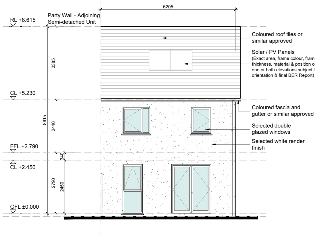
02 Rear Elevation 1:100 @ A3
